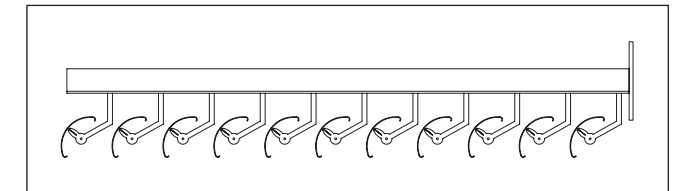
C-lamel Uitkraging tot 1.000 mm. Koker 60 x 40 mm. Uitkraging tot 1.500 mm. Koker 80 x 40 mm.
