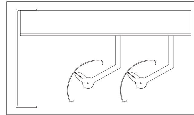
U-profiel 40 x 195 x 40 mm
